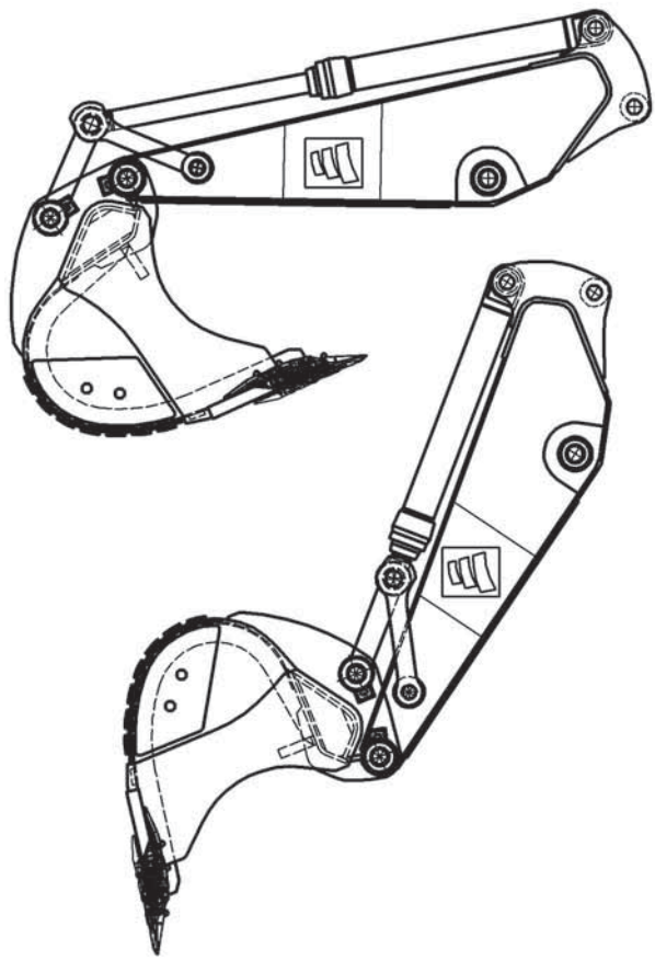
Reißlöffel für CAT 385, Inhalt 5,2 m 3 bei 2100 mm
